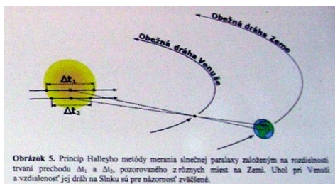
Princip měření Sluneční soustavy, kterou využil i Maxmilián Hella.
